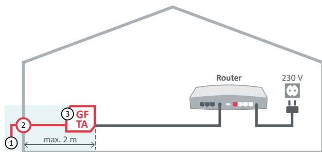
Abbildung 1: Beschreibung Glasfaser-Hausanschluss
